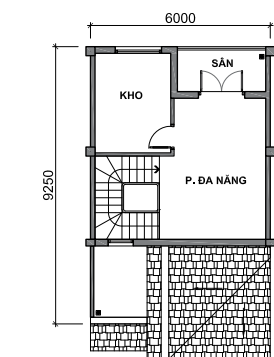
MẶT BẰNG TẦNG 4
