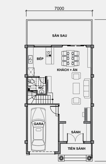
MẶT BẰNG TẦNG 1
