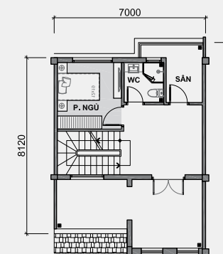
MẶT BẰNG TẦNG 4
