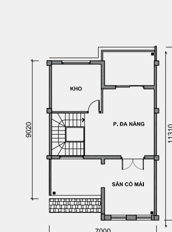
MẶT BẰNG TẦNG 4
