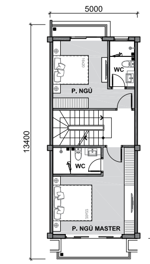
MẶT BẰNG TẦNG 2
