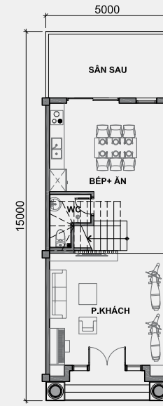
MẶT BẰNG TẦNG 1
