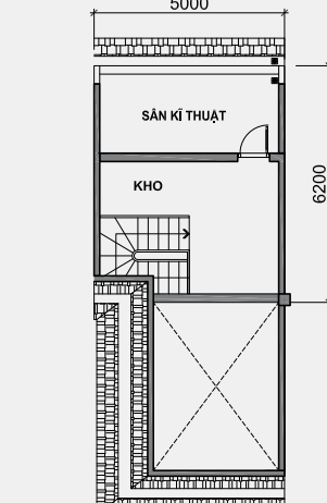
MẶT BẰNG TẦNG TUM
