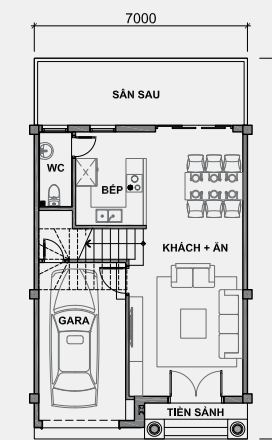
MẶT BẰNG TẦNG 1
