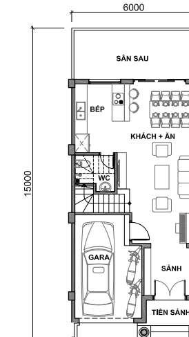
MẶT BẰNG TẦNG 1
