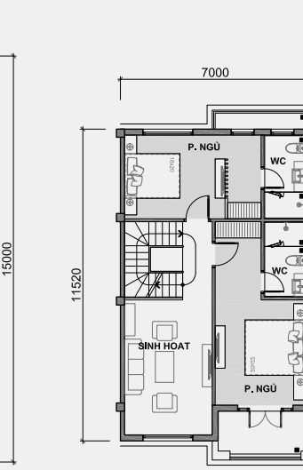
MẶT BẰNG TẦNG 2
