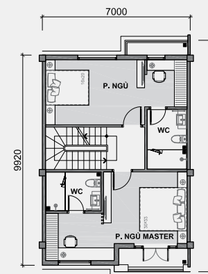
MẶT BẰNG TẦNG 2
